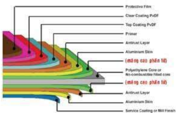
CẤU TRÚC MÀNG CAO PHÂN TỬ ĐƯỢC DÙNG TRONG XÂY DỰNG
